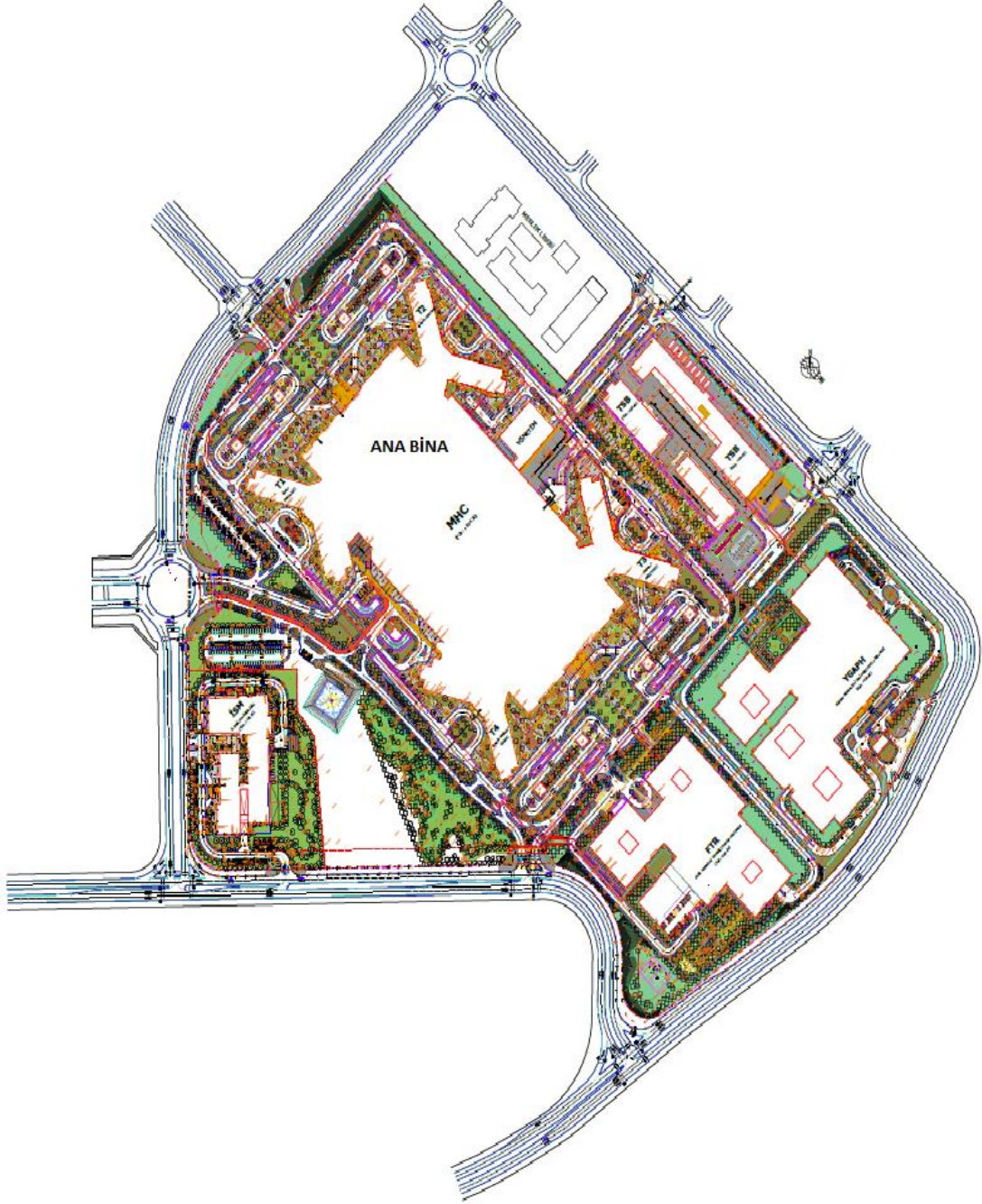
Gaziantep Şehir Hastanesi Yerleşim Planı 1
